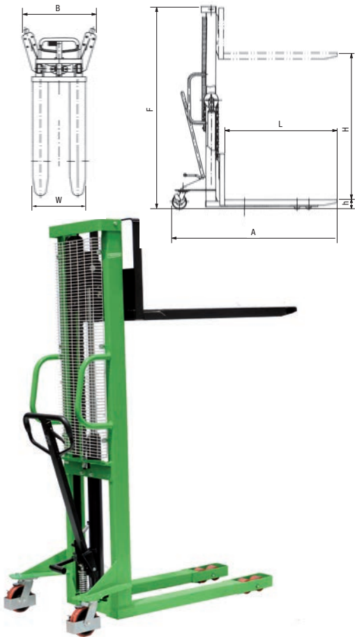
OX55 APILADOR MANUAL 1.000 KG
